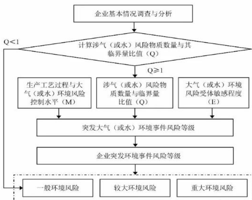
图 2-1 突发环境事件风险评估报告的风险评估程序图
