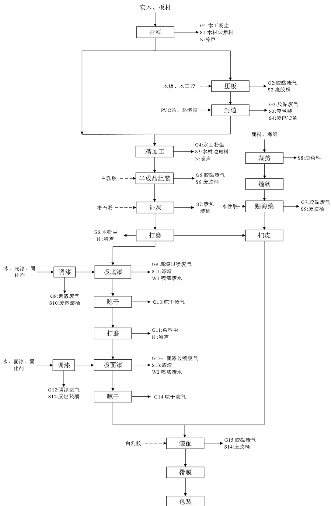
图 1-3 生产工艺流程图
