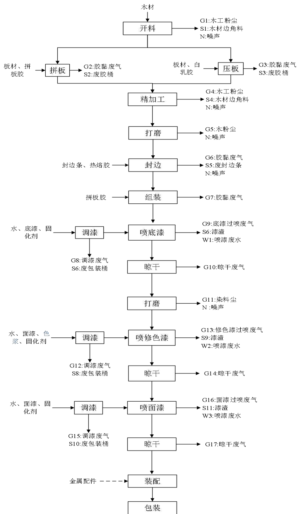
图1-3 生产工艺流程图
