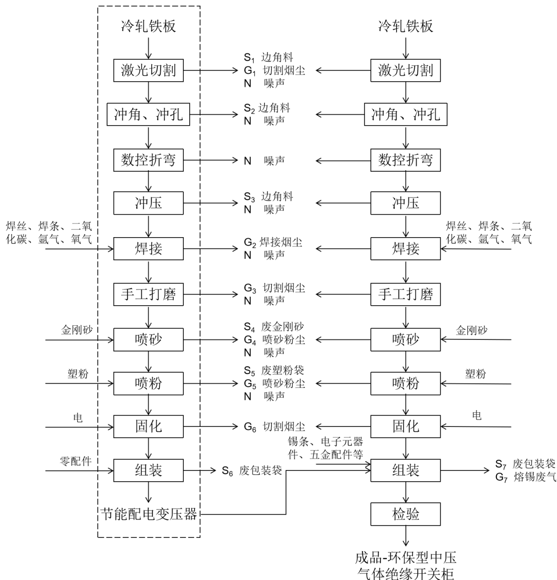
图 3-2 项目生产工艺流程图
