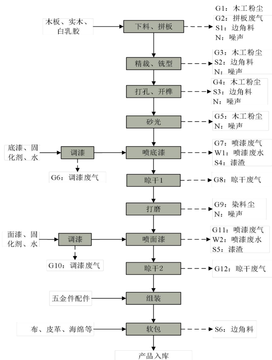
图1-3 生产工艺流程图
