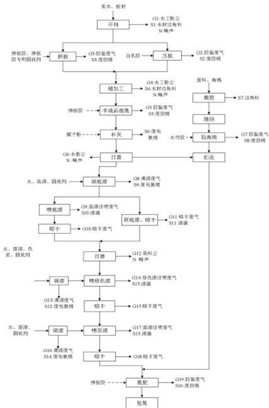
图 3-2 家具生产工艺流程图
